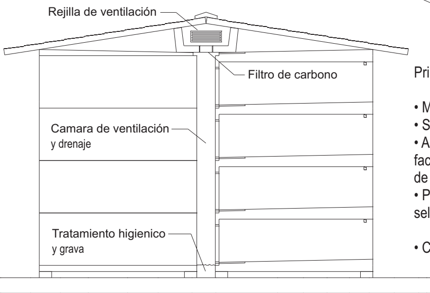
SECCION CONSTRUCTIVA
